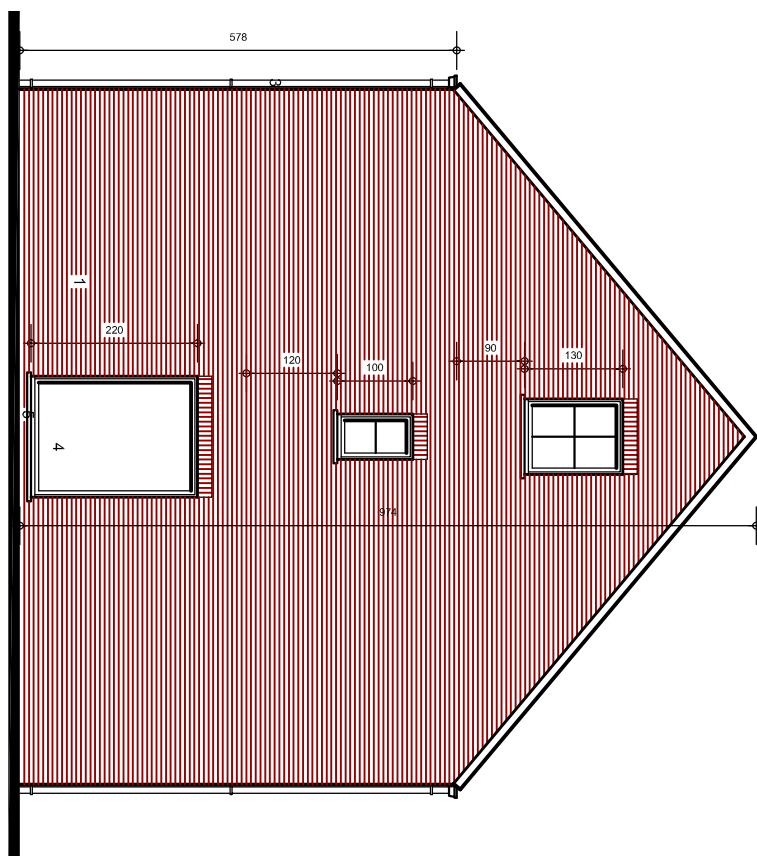
ZIJSGEVEL LINKS
